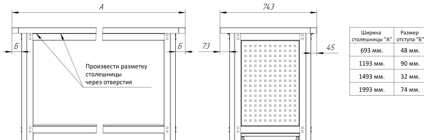
Схема расположения столешницы на раме
